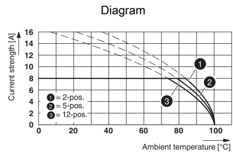
Type: MC 1,5/...-ST-3,81 AU with MC 1,5/...-G-3,81 P... AU THR
