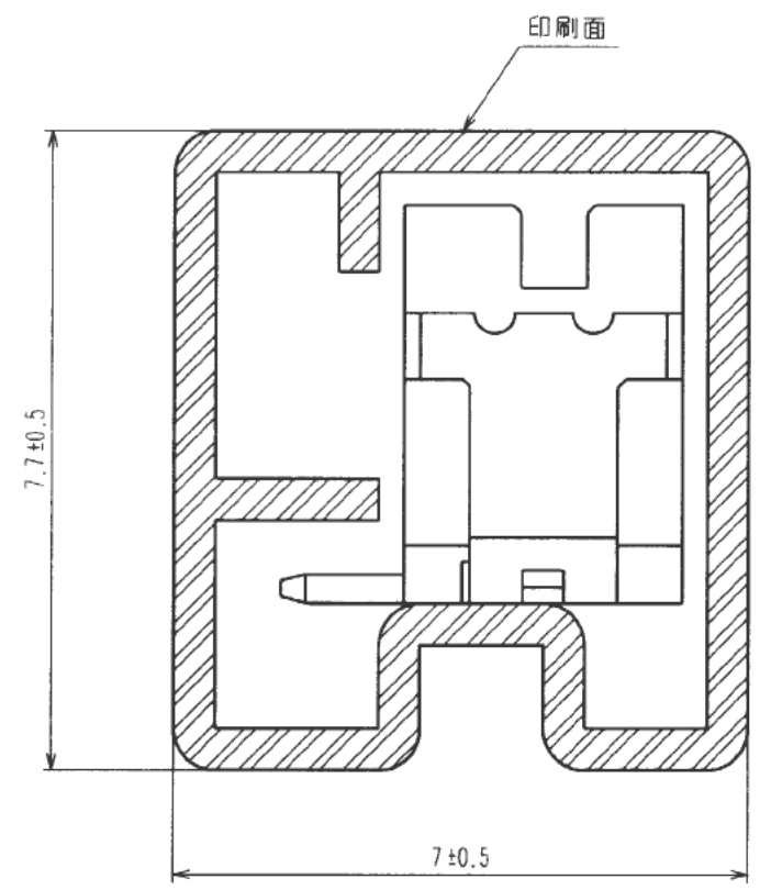
A-A (10:1)
