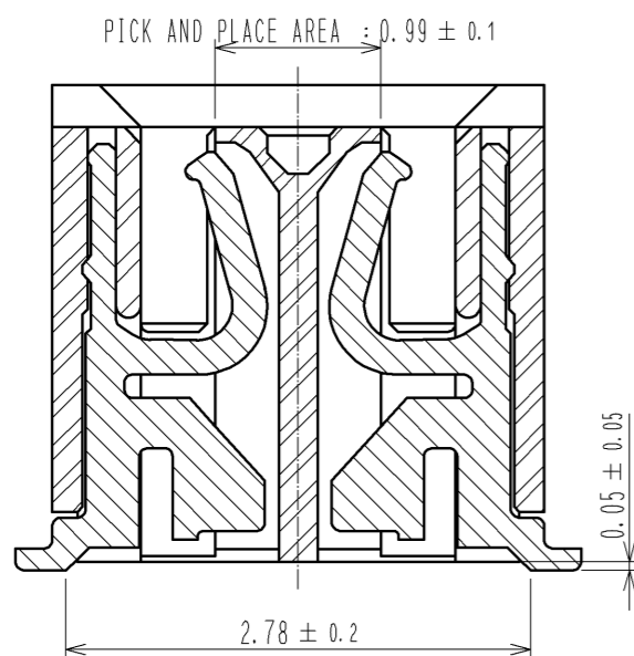
A-A(20:1)
